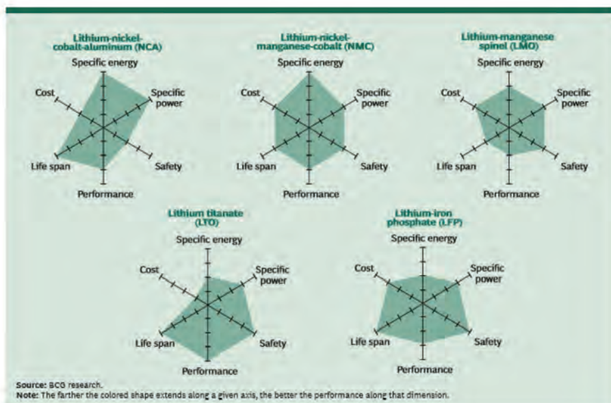
Figura 3: Propiedades de diferentes tecnologías de Li-ion [7]
