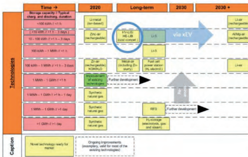
Figura 2: Futuras tendencias en baterías para aplicaciones estacionarias [6]
