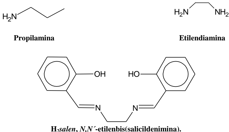
Figura 2. Estructuras de los ligantes propilamina, etilendiamina y H 2 salen.
