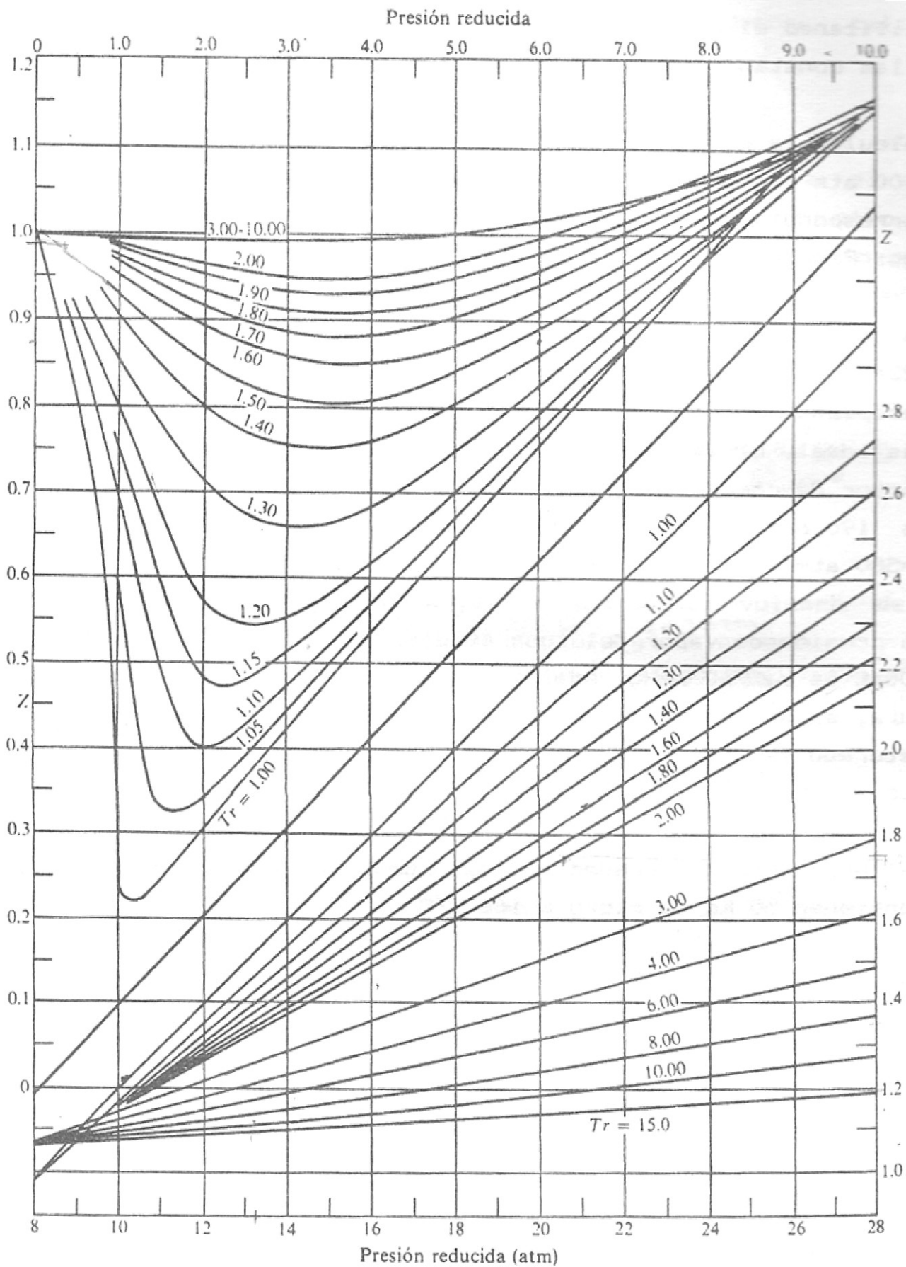
Representación gráfica del factor compresibilidad ( Z ) con respecto a P_r y T_r .
