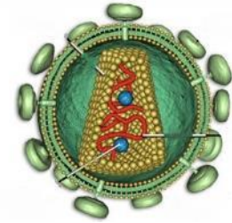
VIH
