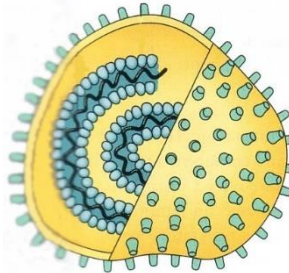
Influenzavirus
