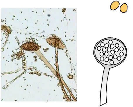
Rhizopus sp
