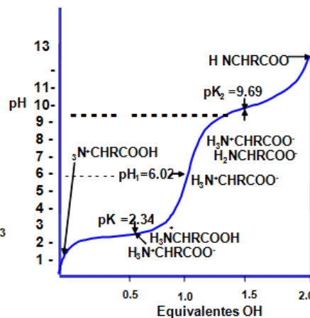
Curva de titulación de la alanina.
