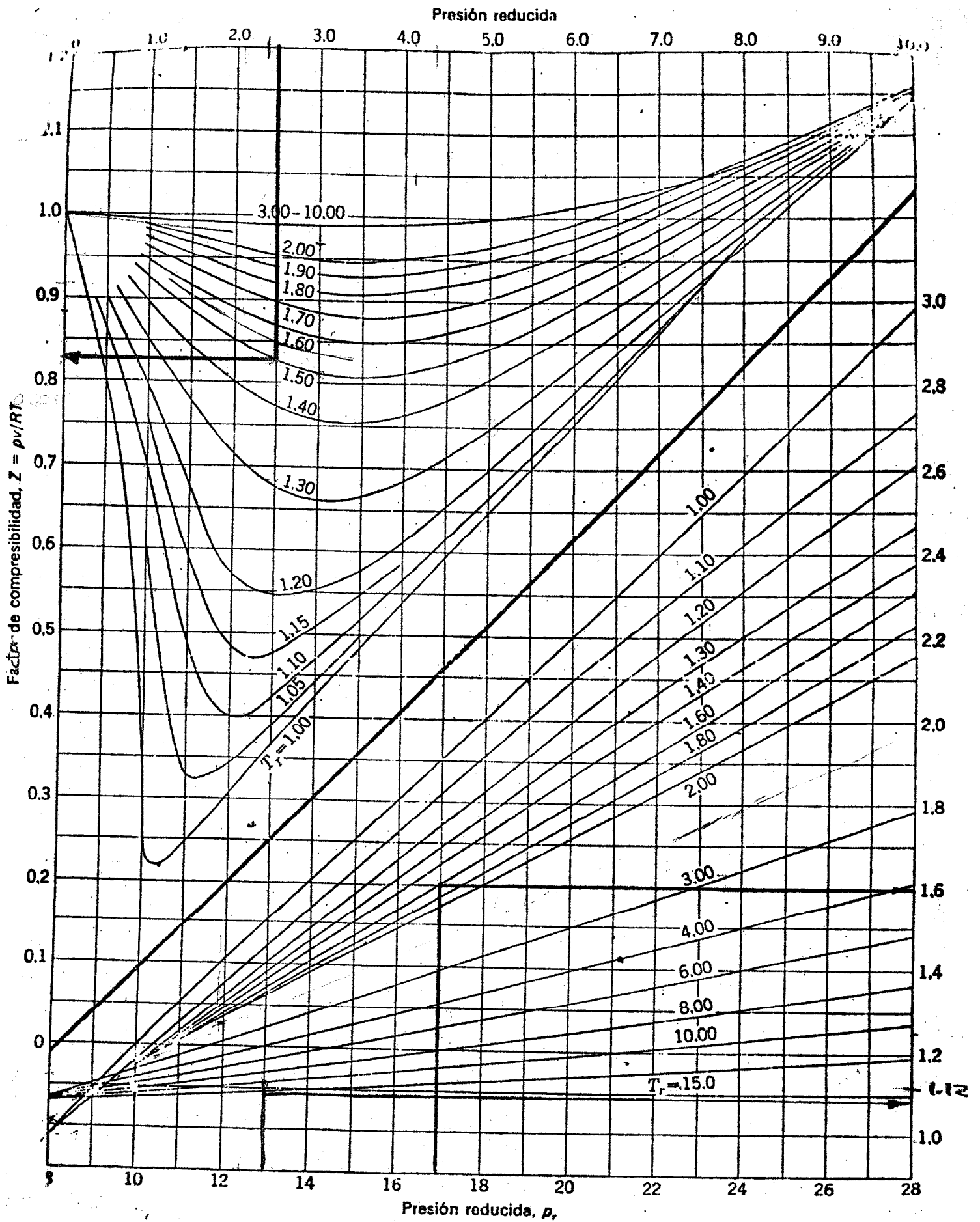
Figura 2-3. Factores de compresibilidad en valores de presión medios y altos. (Basado en datos recogidos por Lydersen, A. L.; Greenkorn, R. A., y Hougen, O. A., Generalized Thermodynamic Properties of Pure Fluids , Univ. of Wisconsin, Eng. Exp. Station, Report 4, 1955. Reproducción autorizada.)
